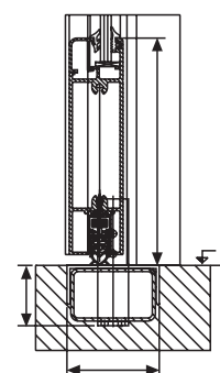
na přání se zápusným podlahovým těsněním
