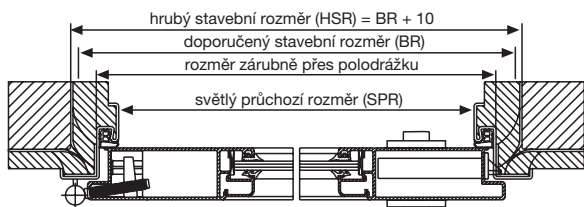
s rohovou zárubní a ornamentálním sklem
