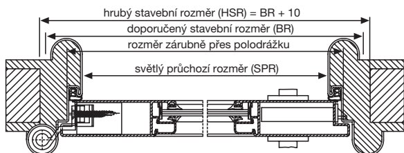
se zárubní typu globus a plnou výplní panelu
