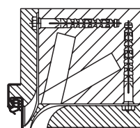
montáž do zdiva kotvy s hmoždinkami
