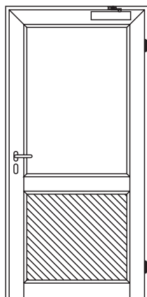
s příčnickem a hliníkovým panelem ve spodní části
