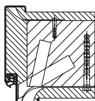
montáž do zdiva kotvy s hmoždinkami
