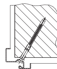
speciální rohová zárubeň montáž skrz dno drážky
