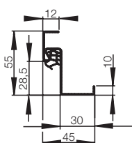
standardní rohová zárubeň
