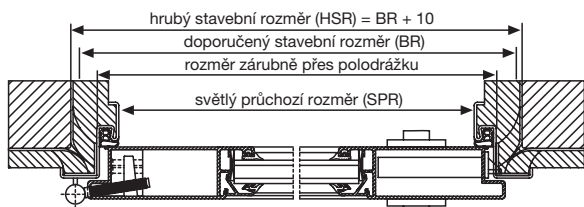
s rohovou zárubní a ISO prosklením
